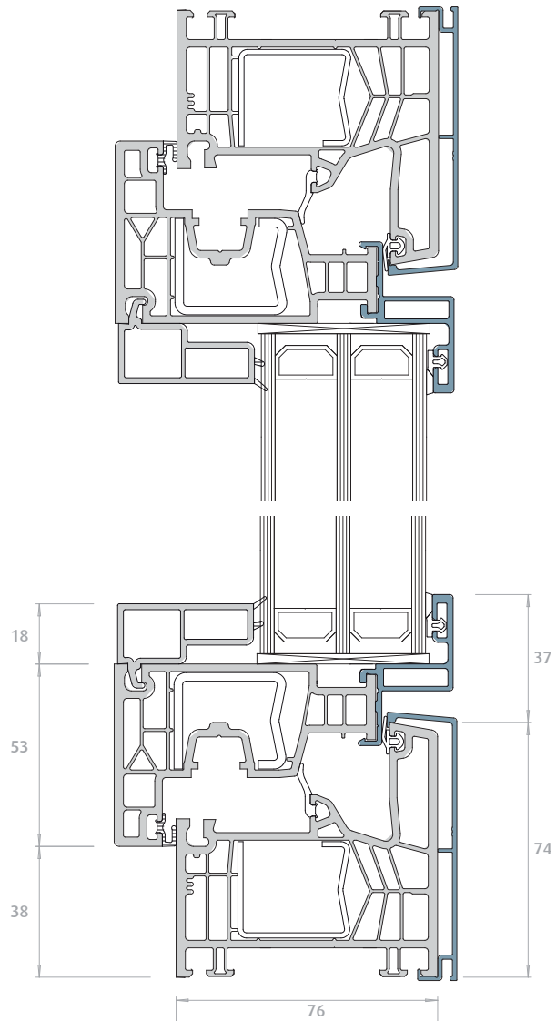
Flügel | Rahmen
