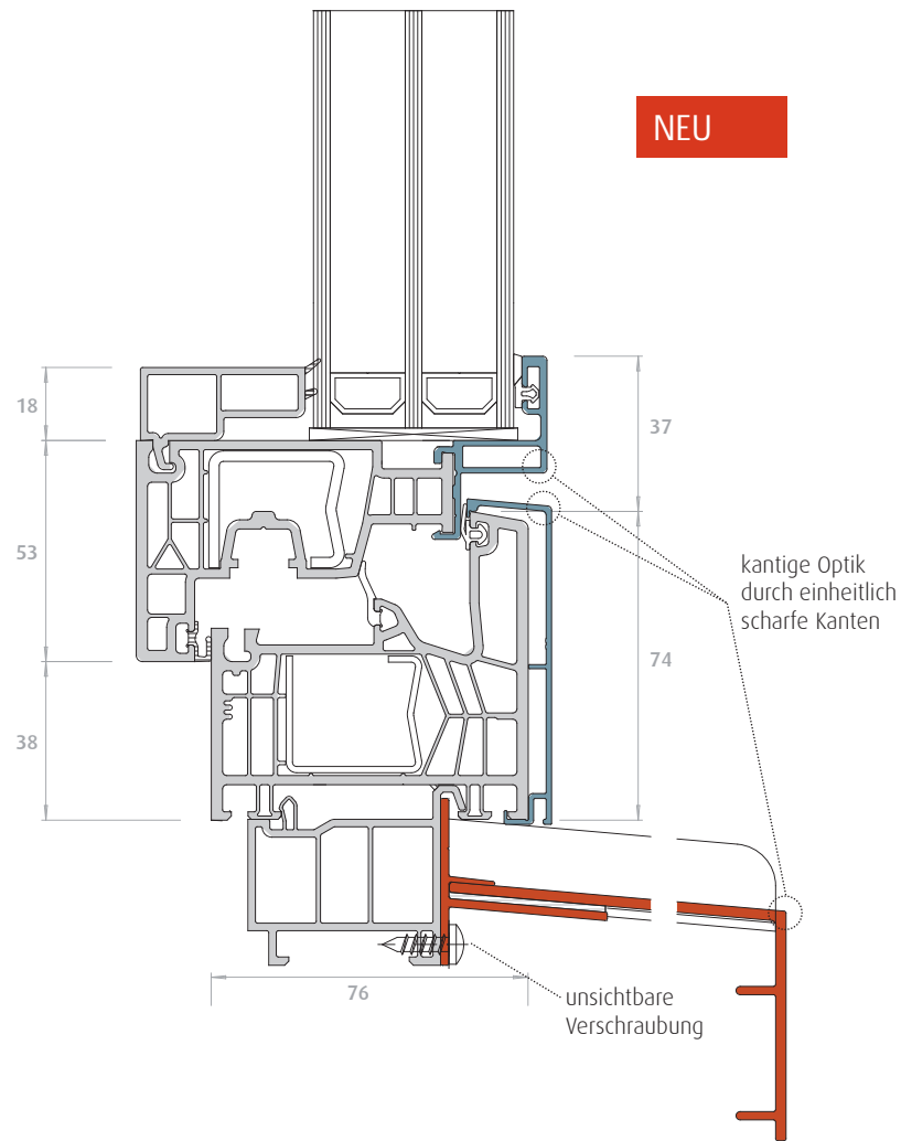
ip-Fensterbank 190 mm Ausladung
